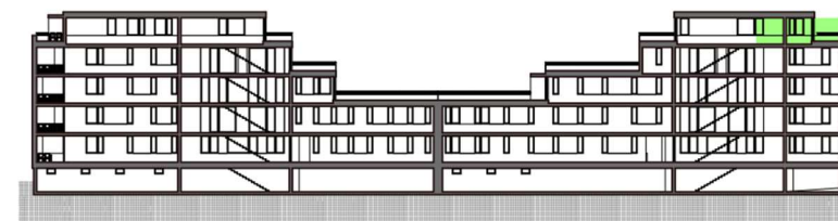
ŘEZ OBJEKTEM
