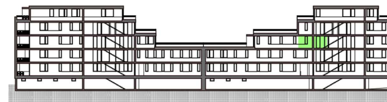
ŘEZ OBJEKTEM
