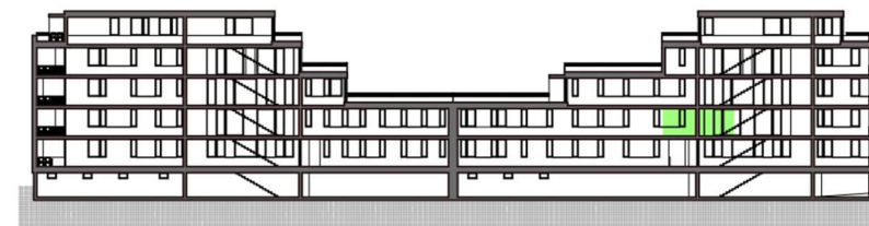
ŘEZ OBJEKTEM
