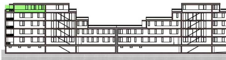
ŘEZ OBJEKTEM
