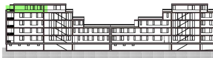
ŘEZ OBJEKTEM
