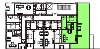
SCHEMA OBJEKTU BD
