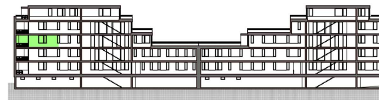
ŘEZ OBJEKTEM
