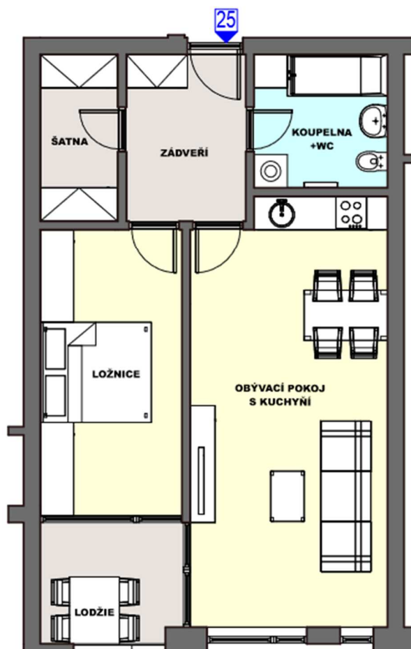
SCHEMA OBJEKTU BD
