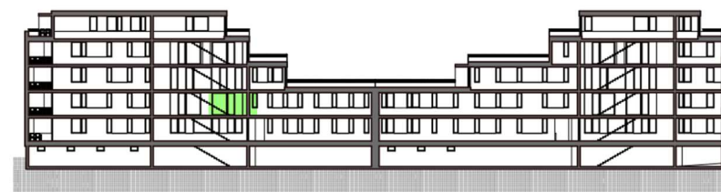
ŘEZ OBJEKTEM
